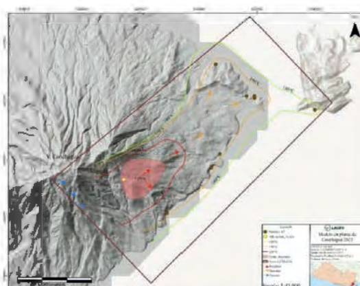
Modelo conceptual en planta del Complejo Volcánico Conchagua
