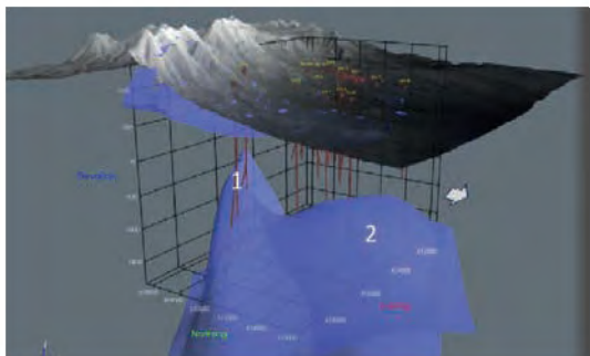
Cúpulas del modelo MT 3D en la zona de Cuyanausul.
