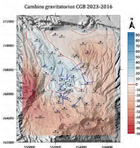
Mapa de cambios gravimétricos entre los años 2023 con respecto al 2016, CG Berlín
